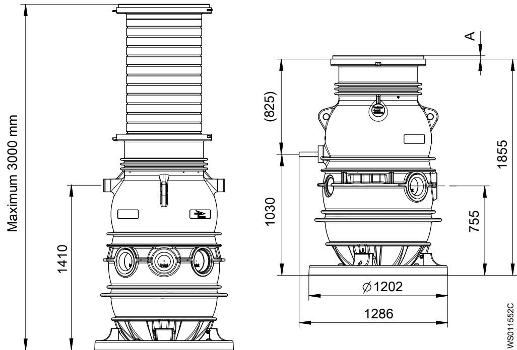
Figur 3: Måttritning. Enhet: mm
