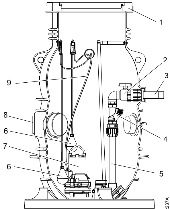
DN50
